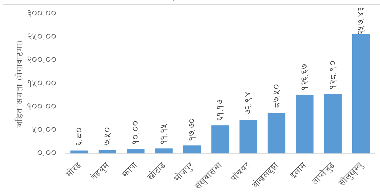
चार्ट ६.१ : जिल्लागत विद्युत उत्पादनको अवस्था (जडित क्षमता)
